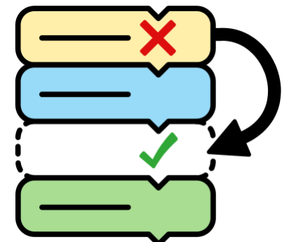
debug
